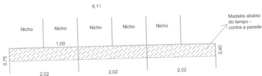
Mesa 01 (maior) - visão lateral
