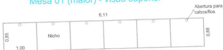
Mesa 01 (maior) - visão superior
