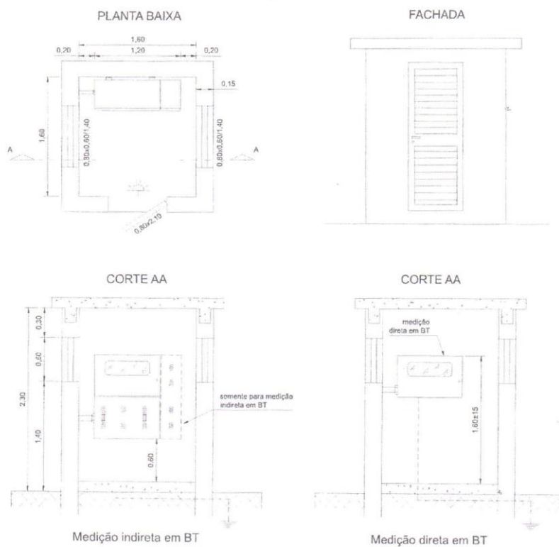
FIGURA 14 - CABINA PARA MEDIÇÃO DIRETA OU INDIRETA EM BT
